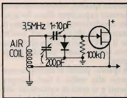
⑤ Questo VFO di W7ZOI è eccezionalmente stabile perché si è usato un minimo numero di componenti di buona qualità. In un secondo momento, si sostituiscono (uno dopo l'altro) i vari componenti e si osserva la variazione della deriva e si effettua l'eventuale compensazione.
