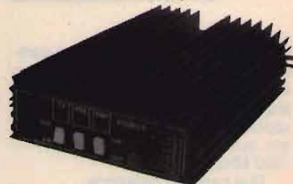
Pramplicatore 25 dB in ricezione Preampifier of 25 dB gain on reception Commutazione elettronica Electronic switch Protezione contro l'inversione di polarità Inversion polarity protection Garanzia 6 mesi escluso transistor finali
