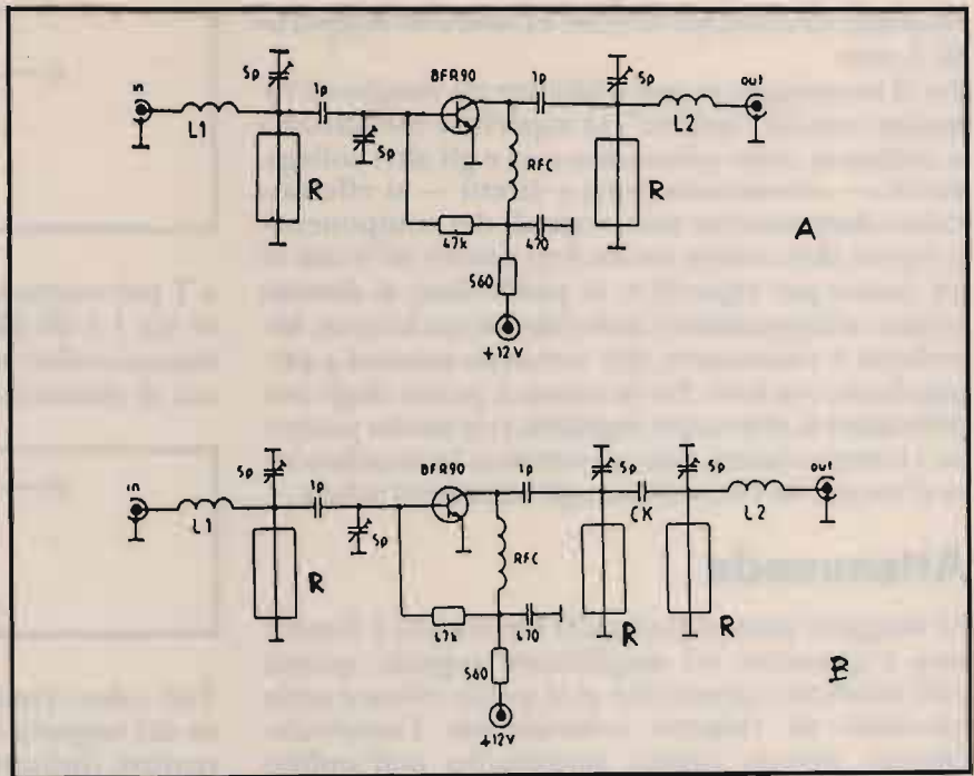
③ Due amplificatori a 1,15 GHz, con risuonatori a perlina di ferrite.
