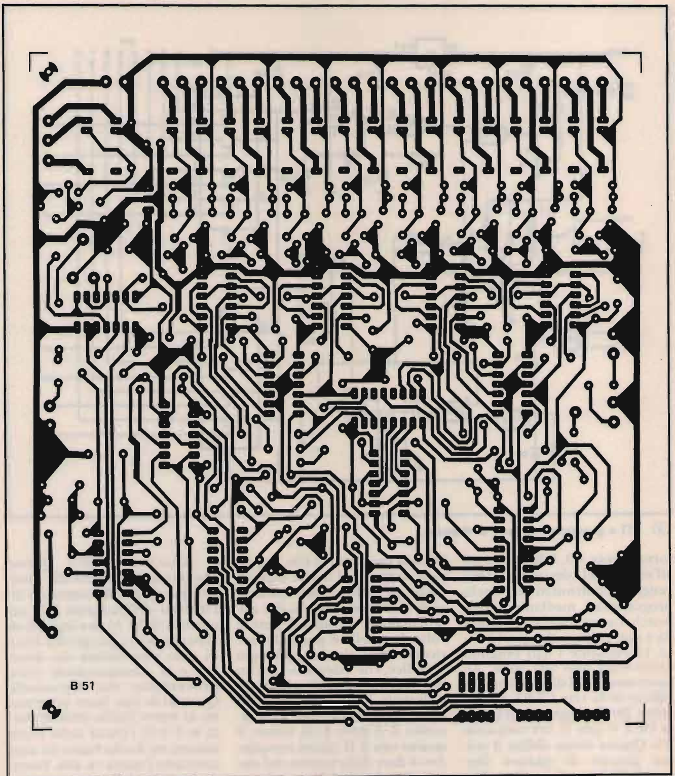
Circuito stampato in scala 1:1.
